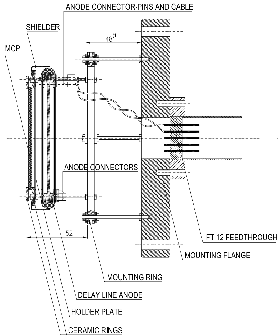
SECTION A-A
